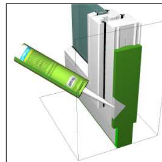
Bild 2: Spritzklotz einfüllen
