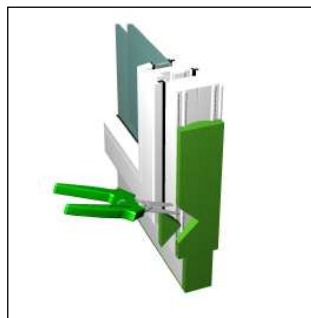
Bild 1: Abdichtung aussparen
